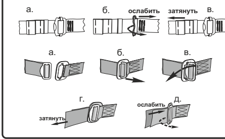
Рис. 9. Соединительно-амортизирующая подсистема
