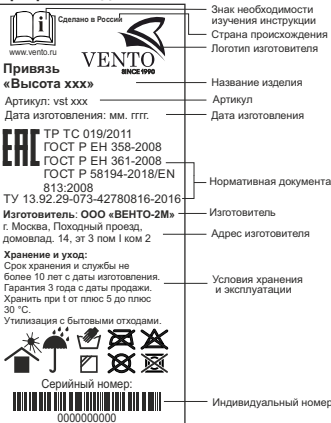
Рис. 3. Маркировка изделия
