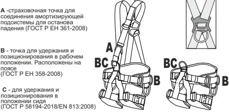
Рис. 2. Типы крепёжных точек
